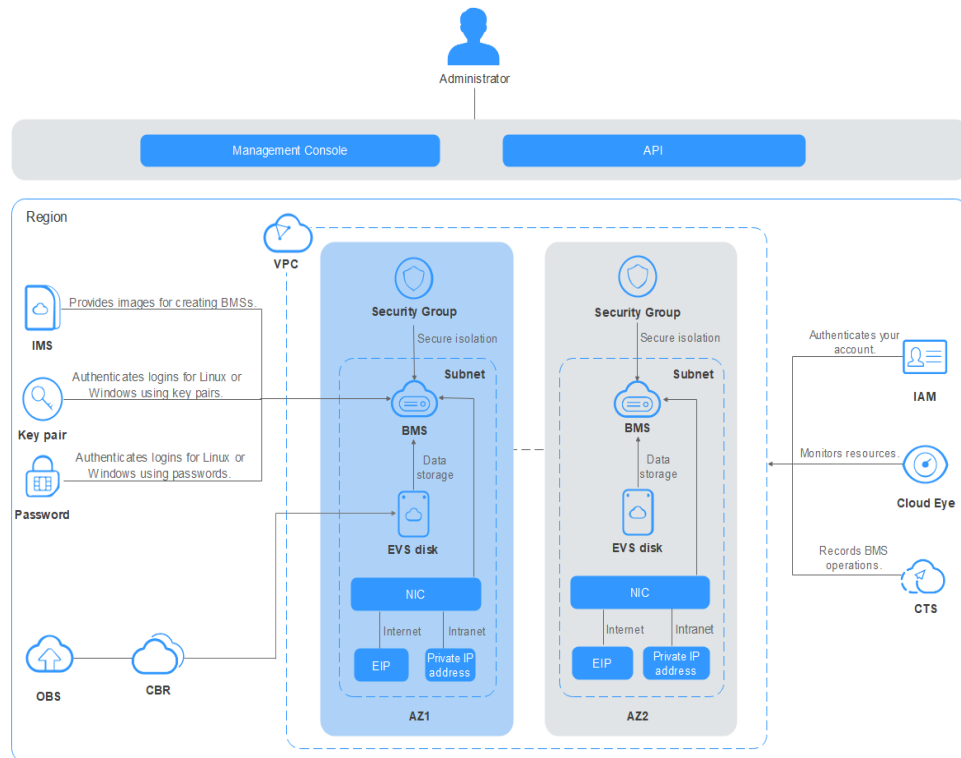
Figura 1-1 Arquitetura do sistema
